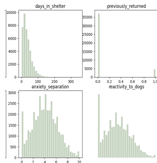
Figura 3.1.2 - Distribución de las variables numéricas principales (Days_in_shelter, Previousuly_returned, anxiety_separation, reactivity_to_dogs)
